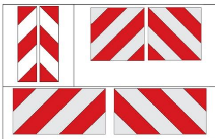
Obr. 9.: Špeciálne označenie širokých vozidiel a vozidiel vykonávajúcich prácu za jazdy.
